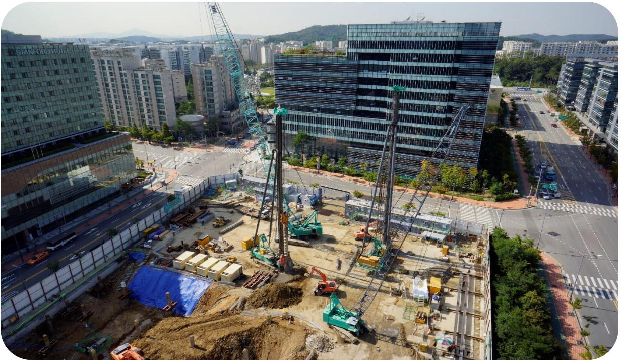
◇ 상암동 삼성 SDS 사옥 신축공사 시공전경 ◇
