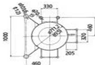
단면 A-A
