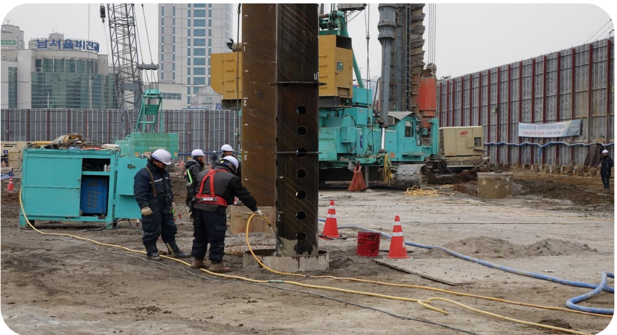
◇ 용인 수지 분당 유타워 신축공사중 CFT COLUMN 근입전경◇
